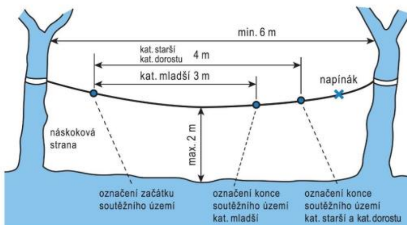
Obr. 5 Brannost - Návrh stanoviště překonání překážky po vodorovném laně
