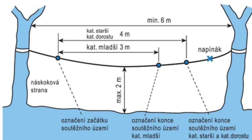
Obr. 5 Brannost - Náskoková strana - Nákres stanoviště překonání překážky po vodorovném laně
